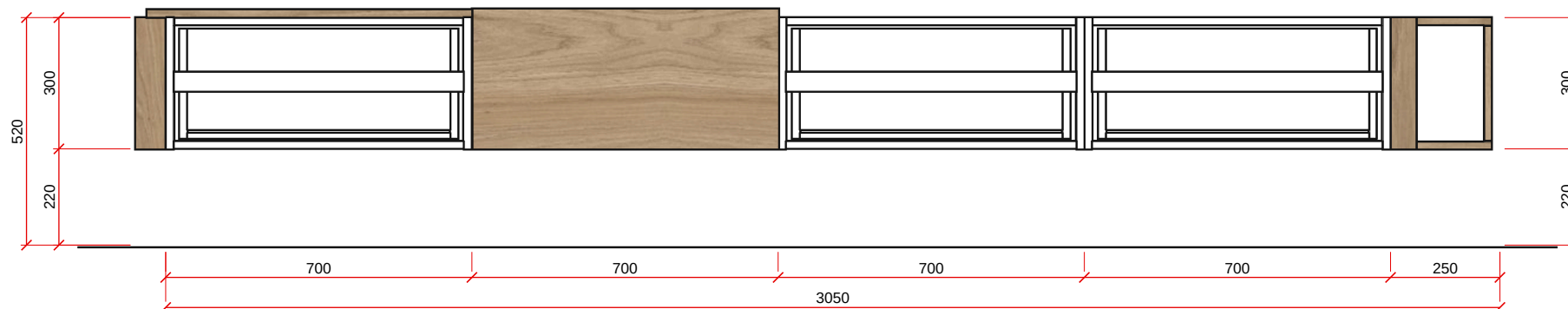
VISTA A - ESC. 1:15
